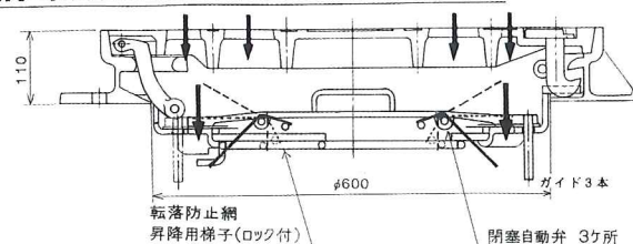
SOGO-6-B型荒目 (防臭)
