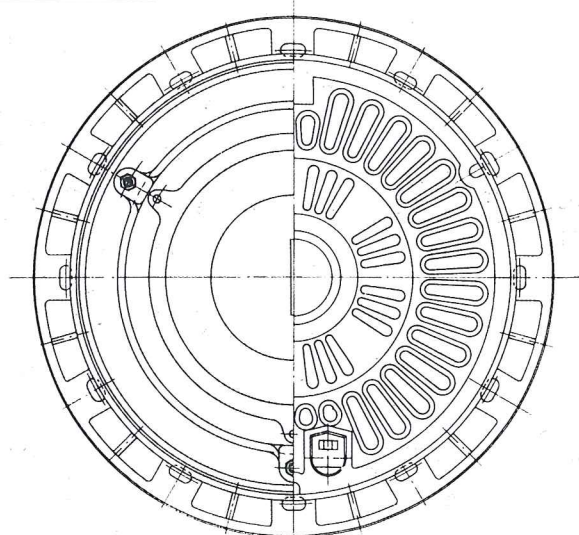
SOGO-6-A型荒目 (簡易防臭)
