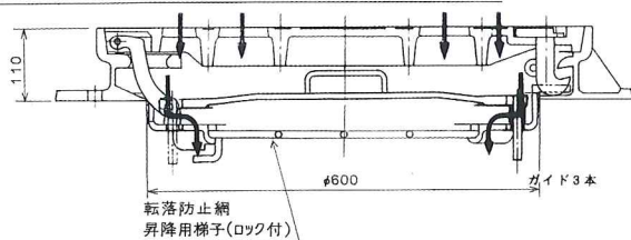
SOGO-6-A型荒目 (簡易防臭)
